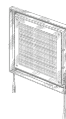
Manuelle Einstellung des freien Querschnitts (R)
