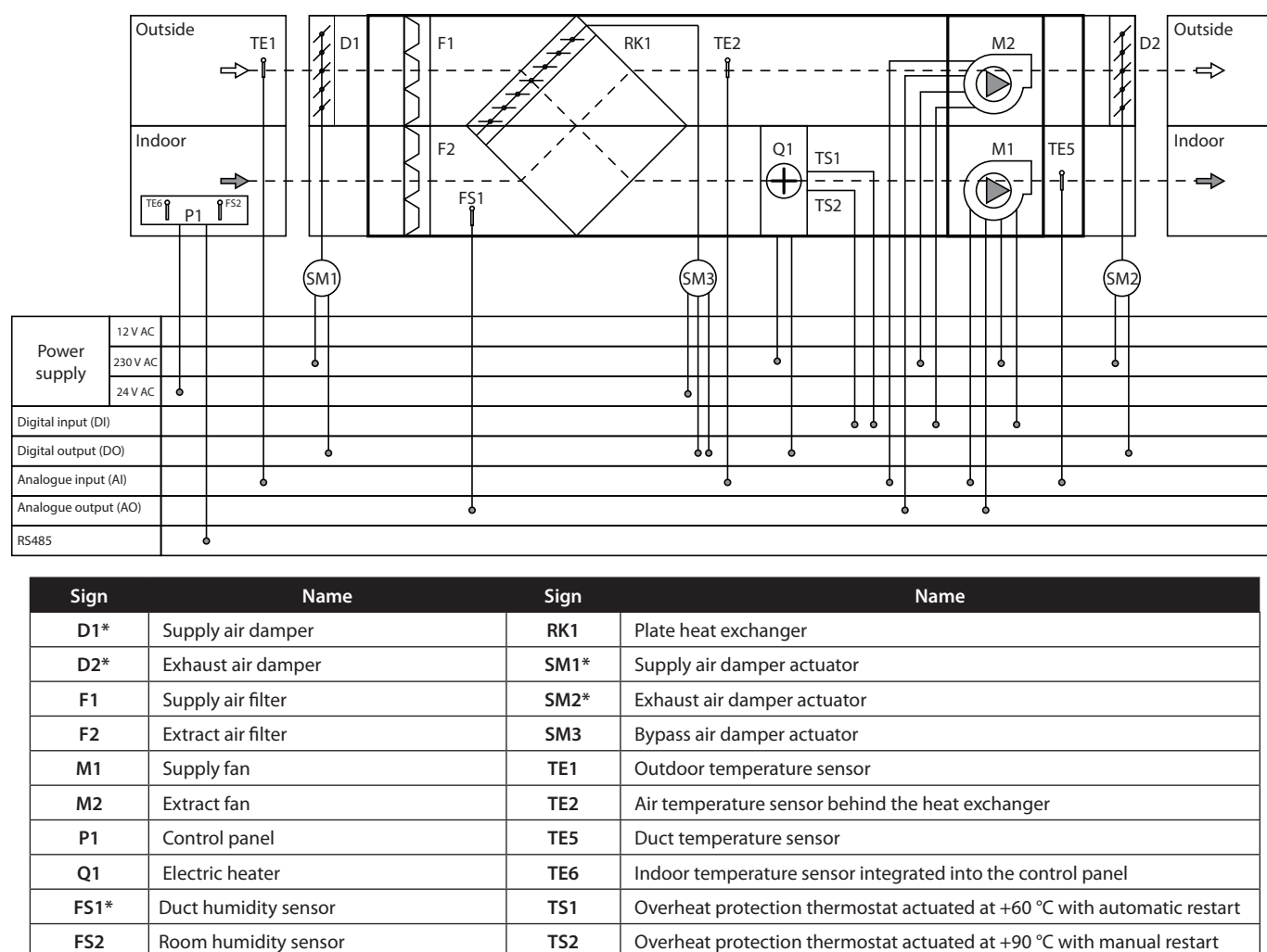
Fig. 11. KOMFORT EC DE2000-12 ... EC DE4000-21 wiring diagram
