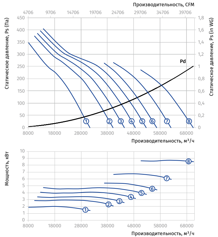
Типоразмер: 1120 Количество полюсов: 6
