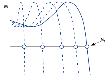
График крутящего момента при пуске от ПЧ
