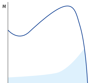
График крутящего момента при прямом пуске
