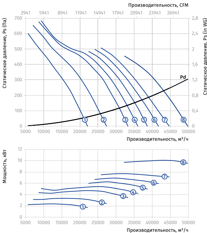
Типоразмер: 900 Количество полюсов: 4
