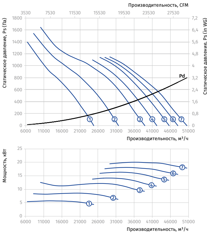
Типоразмер: 710 Количество полюсов: 2
