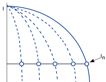
График тока при пуске от ПЧ
