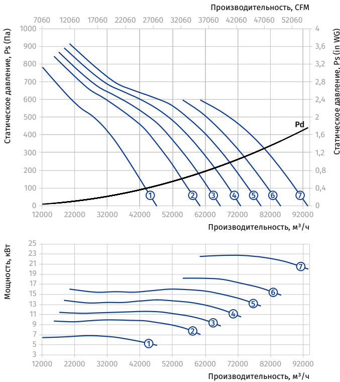
Типоразмер: 1120 Количество полюсов: 4
