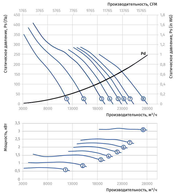
Типоразмер: 710 Количество полюсов: 4
