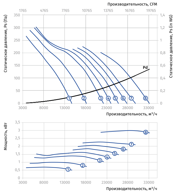
Типоразмер: 900 Количество полюсов: 6
