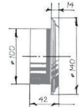
Круглая решетка
