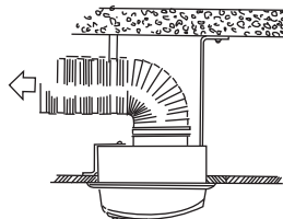
Deckenmontage mit Montagewinkeln
