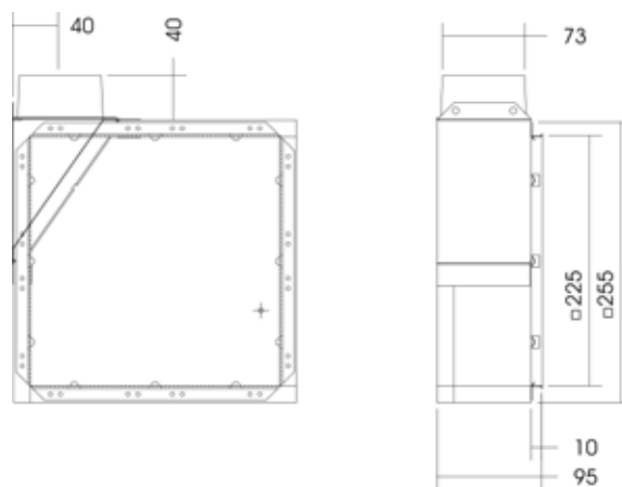
Unterputzgehäuse BF
