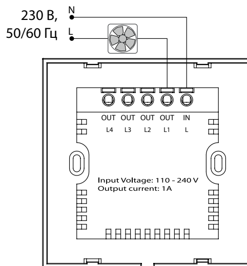
Схема электрических соединений (только для SGS E1)
