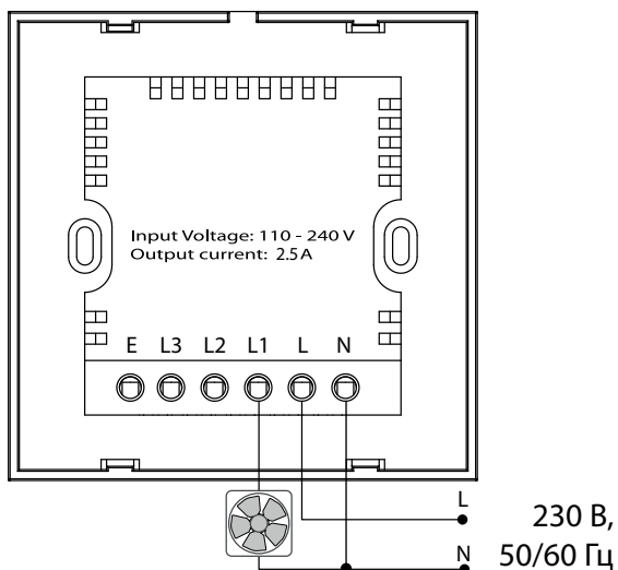
Схема электрических соединений (SGS E1 и SGS E2.5)
