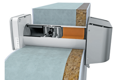
Montagebeispiel mit Haube für dünne Wände AH-S grau 160 / AH-S chrome 160
