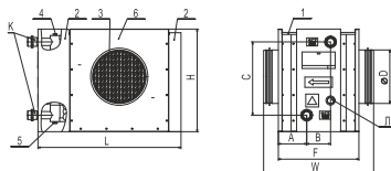
рисунок 2 Основные размеры WKH с подсоединением к круглому воздуховоду
