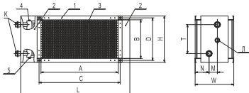
рисунок 1 Основные размеры WKH с прямоугольным подсоединением к воздуховоду
